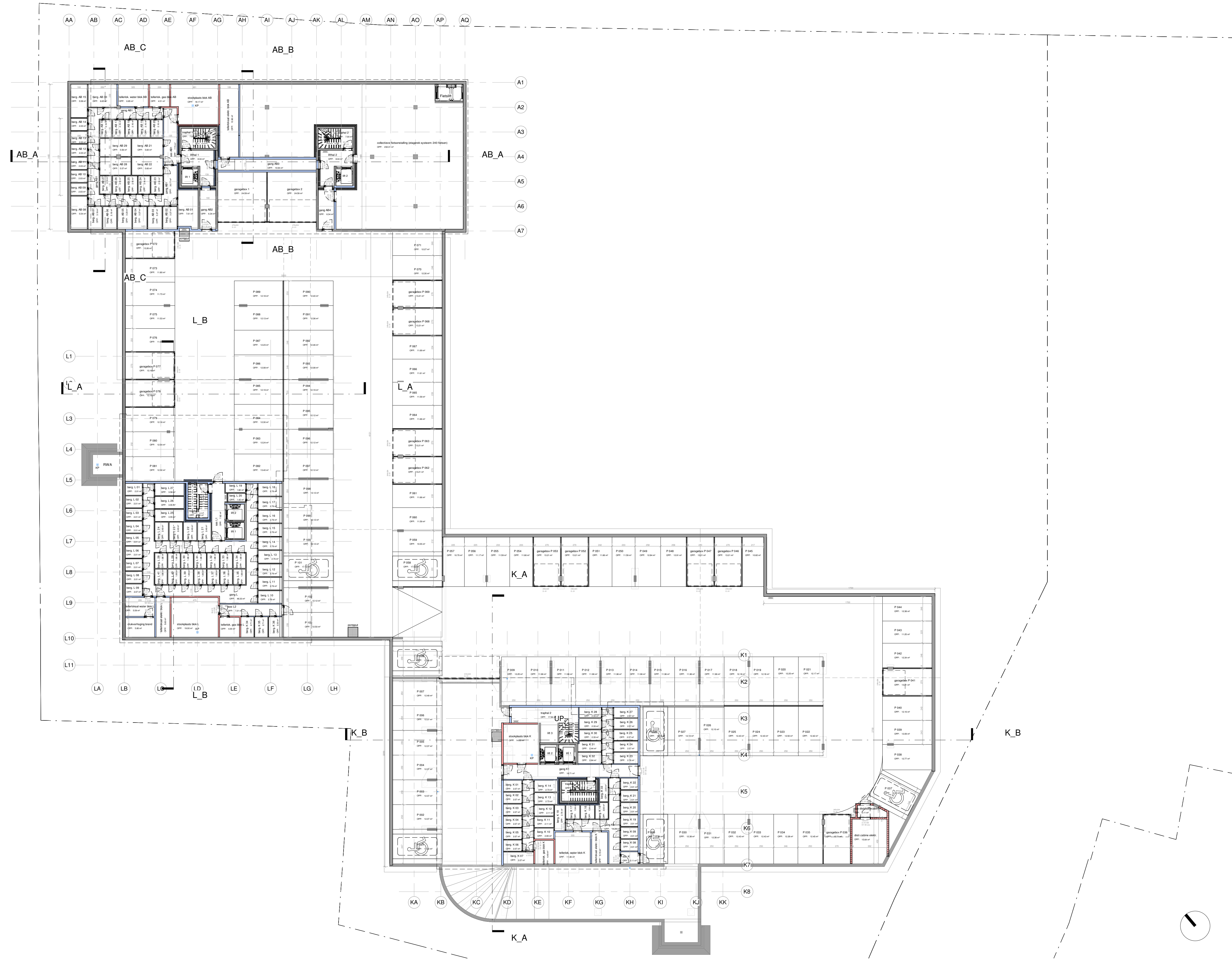
Grondplan parkeergebouw -01
